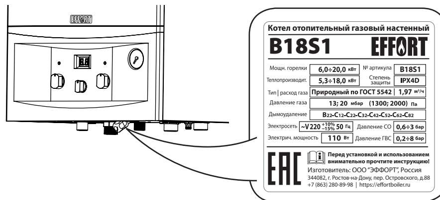
Расположение шильдика котла
